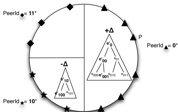
(b) Après le rafraîchissement, tous les pairs de e'_{10} et e'_{100} ont mis à jour leur arbre de fragmentation. Les pairs de e'_{11} ne connaissent pas la valeur \Delta utilisée.
