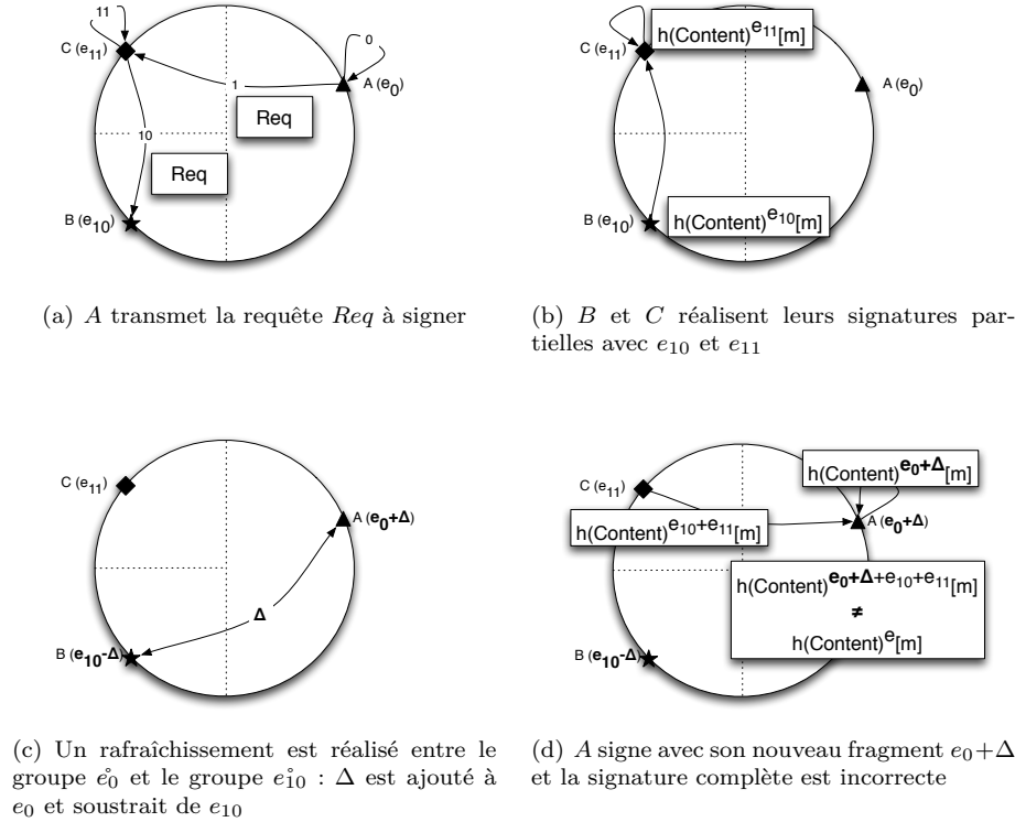
FIGURE 4.5 – Concurrency entre un rafraîchissement et un processus de signature distribuée. La signature finale est incorrecte, bien que tous les participants soient honnêtes.
