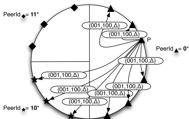
(a) P transmet la requête de rafraîchissement contenant l'identifiant de sa feuille locale 001, l'identifiant de la feuille distante 100 et la valeur aléatoire \Delta . Chaque pair retransmet également cette requête (non illustré ici pour des raisons de lisibilité).
